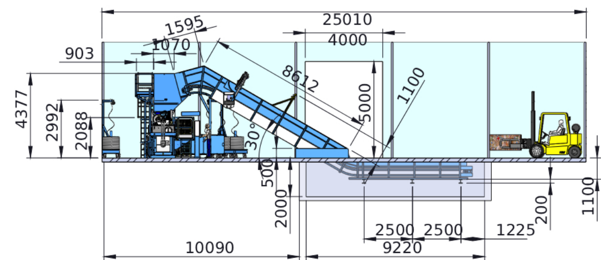
COUPE C-C
