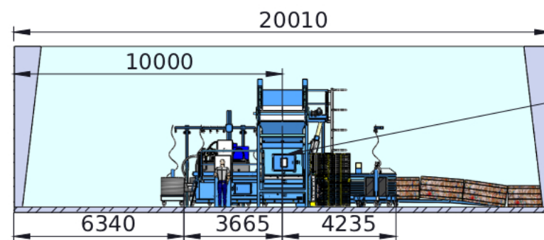
COUPE D-D
